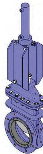
С гидроцилиндром
